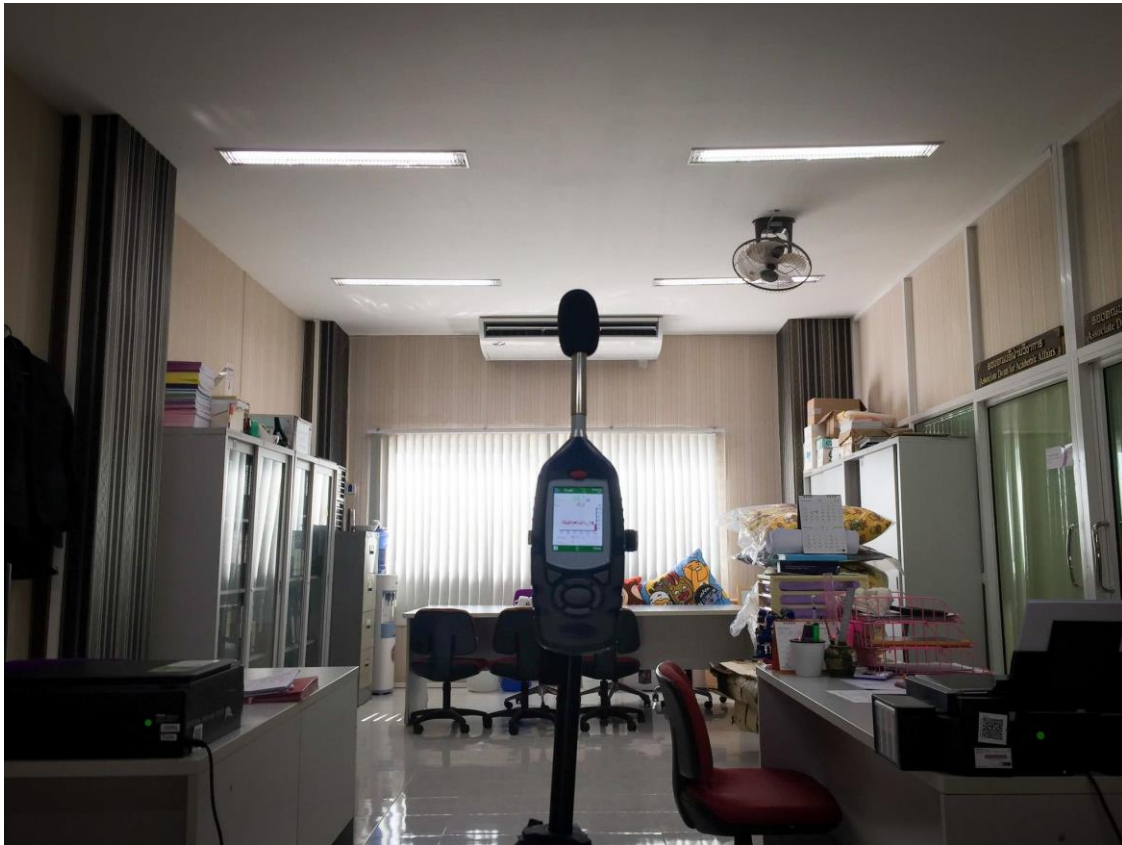
การตรวจวัดระดับเสียงภายในสำนักงานคณะนิติศาสตร์ ห้อง A303
